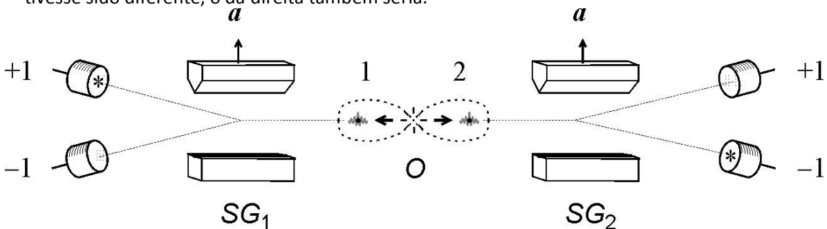
Fig. 3. Ilustração da anticorrelação perfeita exibida pelo estado de singlete.
