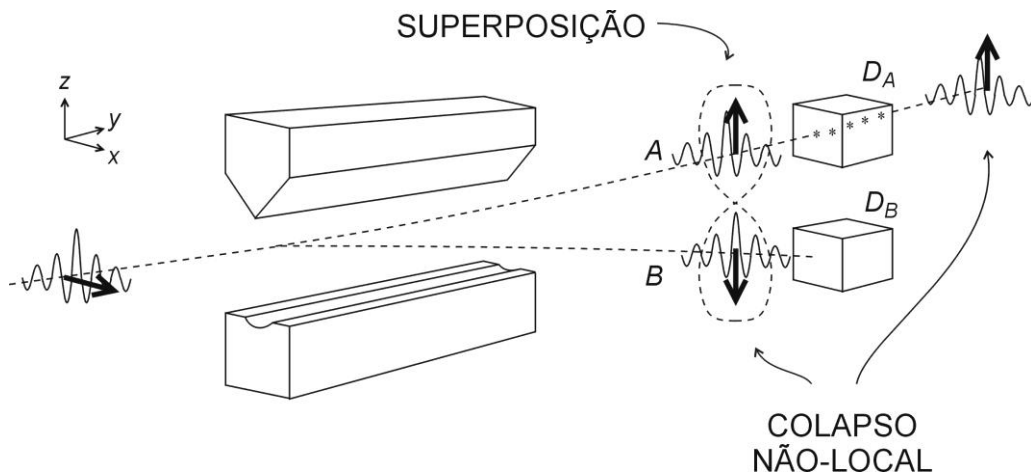
Fig. 1. Superposição e colapso no experimento de Stern-Gerlach.
