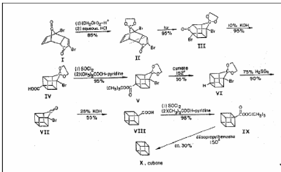
Figura 1. Ecuaciones de reacción para la síntesis del cubano. En cada flecha se incluye el reactivo necesario para lograr la transformación y el rendimiento obtenido. Cada uno de los nueve pasos involucra de entre cinco a veinte procedimientos diferentes: pesado, disolución, mezclado, calentamiento, separación y caracterización analítica (Garritz, 1999).
